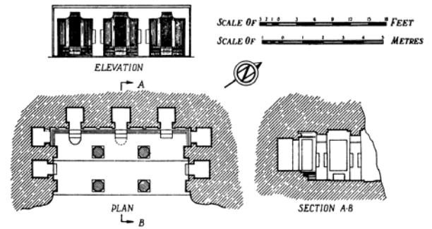
図 13. カルマンガカム石窟平面図、断面図、立面図
