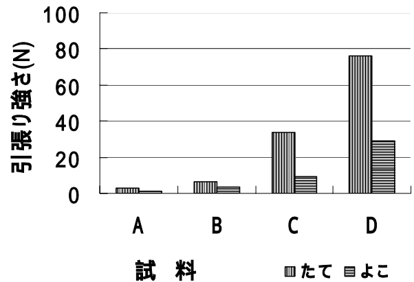
図 1 各試料における引張り強さ
