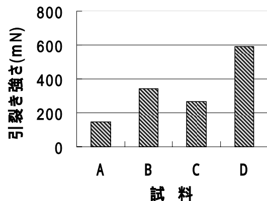
図 2 引裂き強さ
